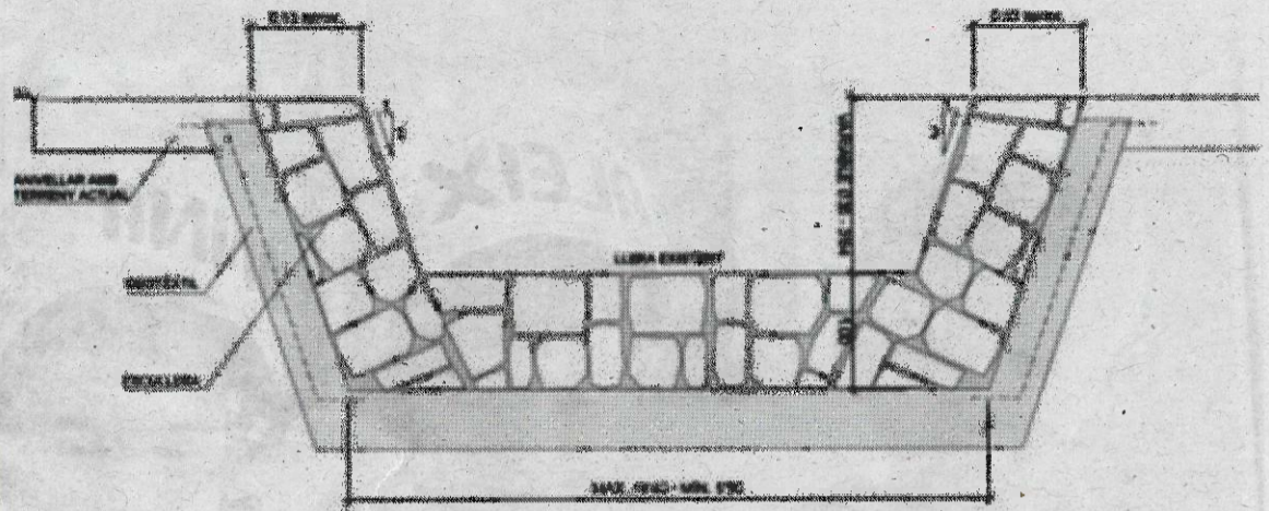
SECCIÓ AMB ESCULLERA ESCALA 1:50
